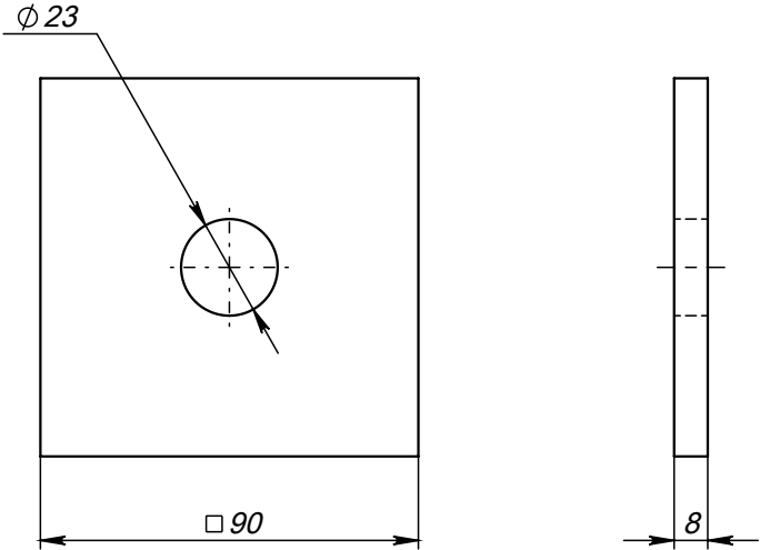
Поз.3 (Плита)
